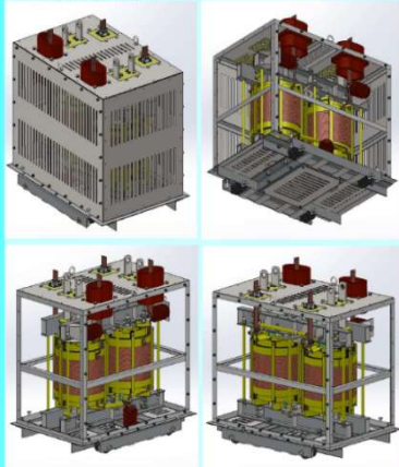
Трансформаторы однофазные вольтодобавочные для сетей 6 и 10 кВ с питанием от сети 380 В
