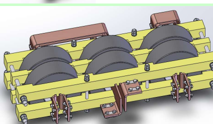
а, в, с – входные вводы уравнителя; А, В, С – выходные вводы уравнителя.
