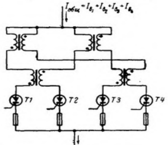
Рис. УП-2 Выравнивание токов в двух переменного соединенных тиристорах с помощью четырех реактивных катушек.
