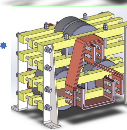
а, в, с – входные вводы уравнителя; А, В, С – выходные вводы уравнителя.
